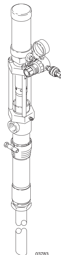
Pumpe mit einstellbarer Länge zur Spundlochmontage
